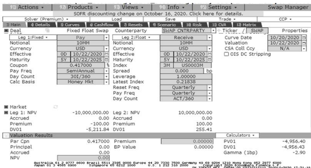
圖二：美國付固定利率 5 年期利率交換合約利率風險特性
